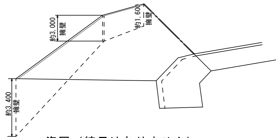
姿図（縮尺はありません）
