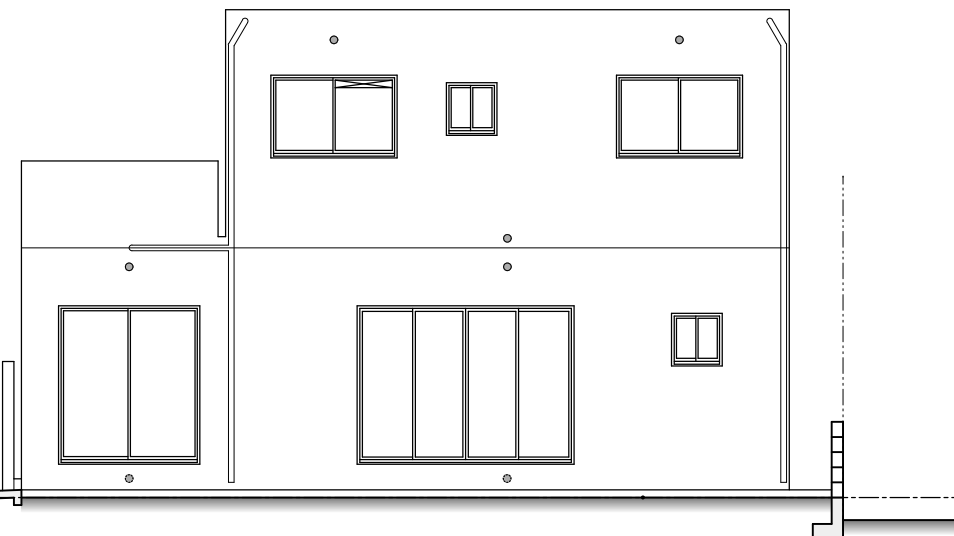
西側立面図
