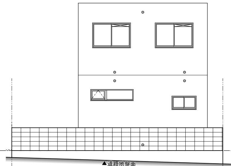
南側立面図
